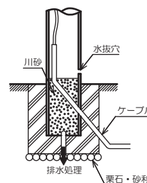
コンクリート基礎の場合
