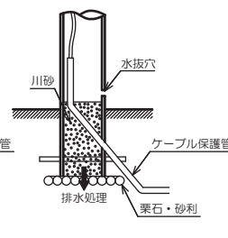
植栽への施工の場合
