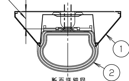
断面詳細図
