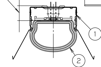
断面詳細図
