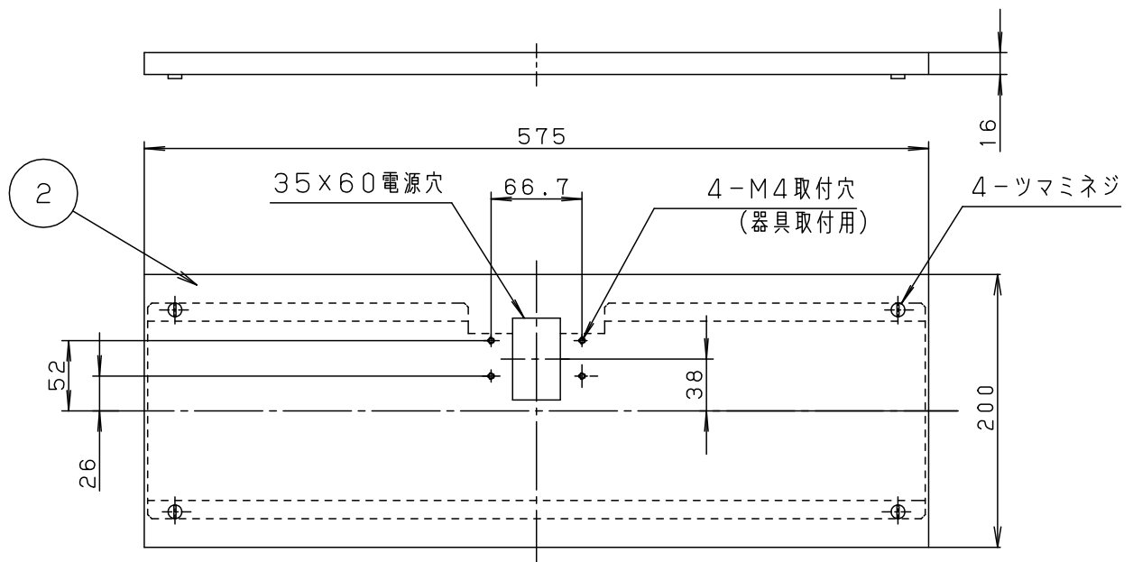
背面図
