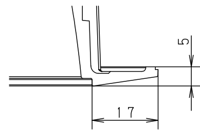
枠部詳細
