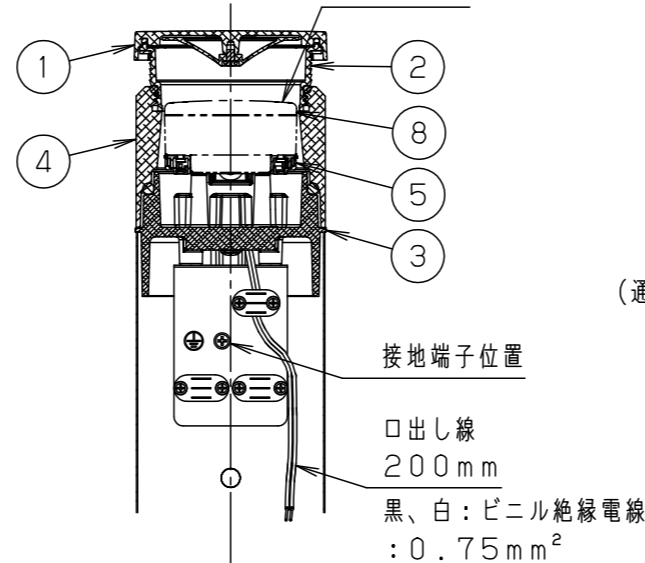
灯具部詳細図 (S=1:4)
