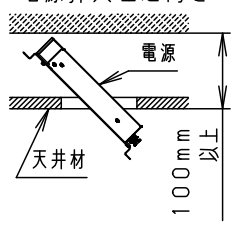
電源挿入埋込高さ
