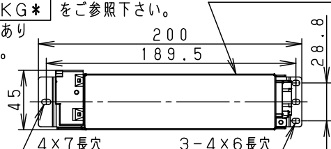
LED電源ユニット
