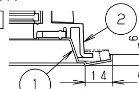
調光信号線用端子 (送り可能)
