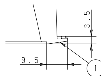
杵部詳細
