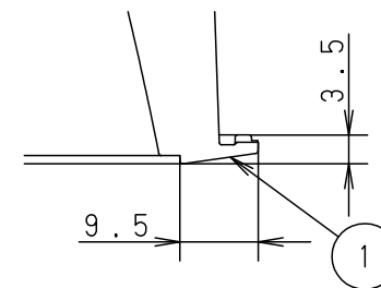
枠部詳細
