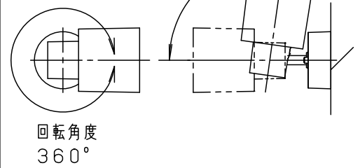
可動範囲
