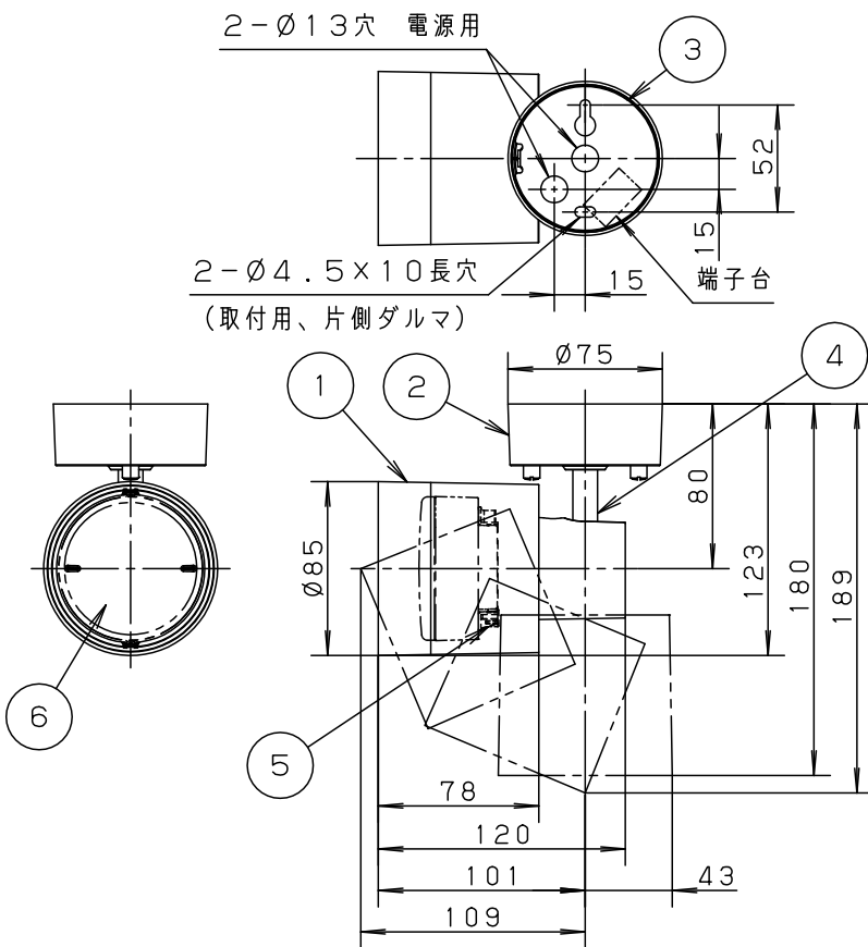
可動範囲
