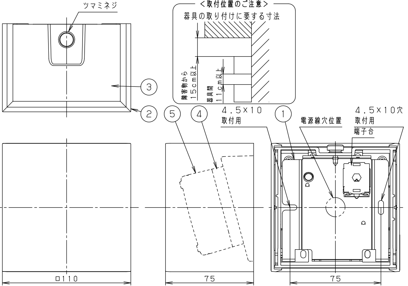
(背面図)
