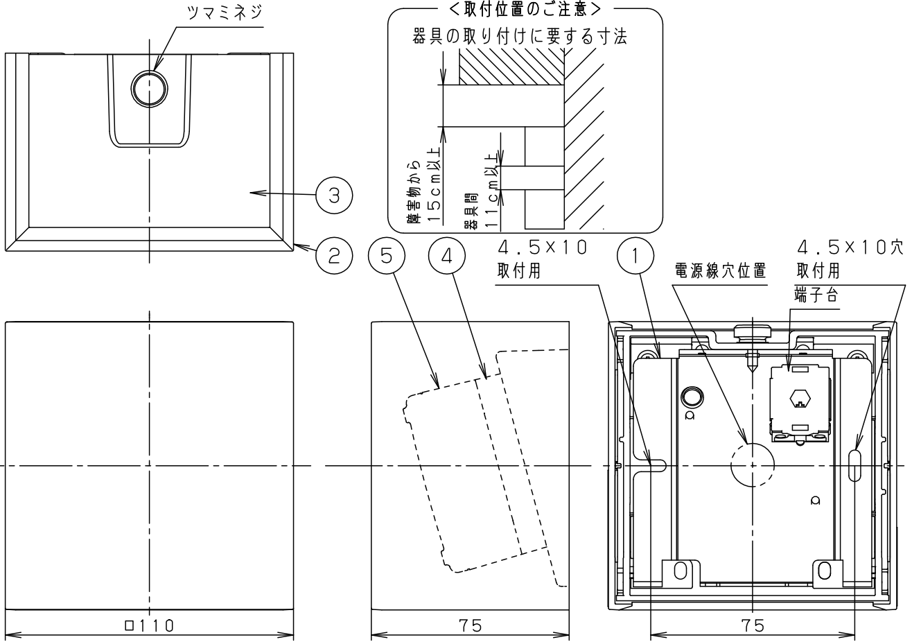
(背面図)
