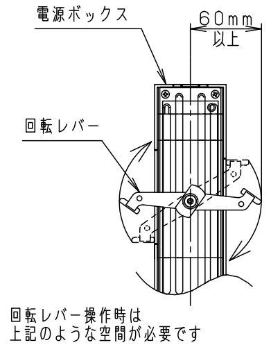
器具施工時必要寸法
