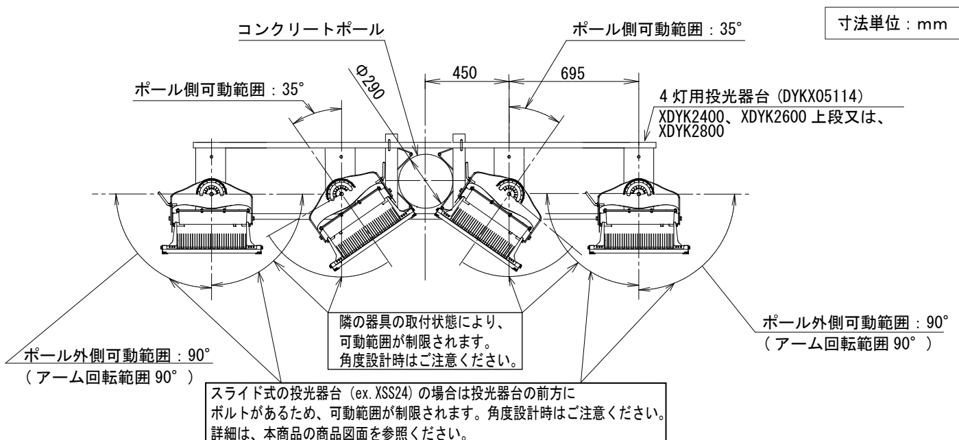
図3 投光器台に取り付け時の注意事項
