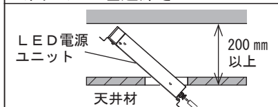
<図1> 埋込深さ
