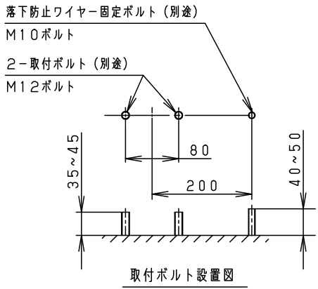
取付ボルト設置図
