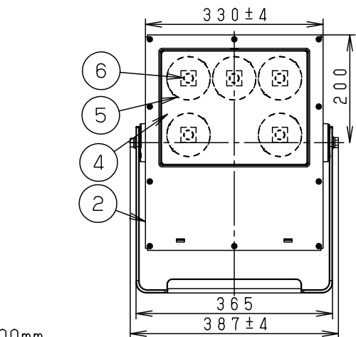
電源線 器具外500mm (ビニルキャプタイヤケーブル 3芯 1.25mm 2 )
