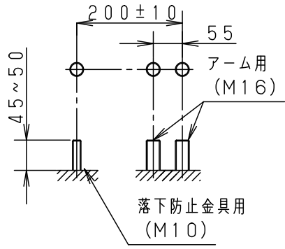
取付ボルト設置図
