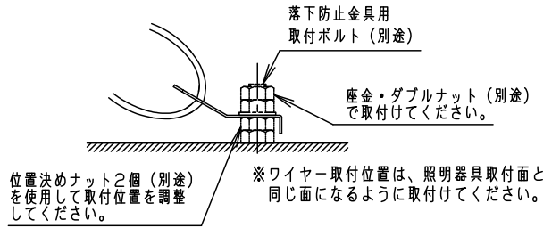
落下防止金具部
