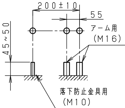
取付ボルト設置図
