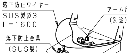
落下防止ワイヤー取付図
