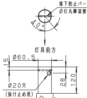
適合ポール先端形状
