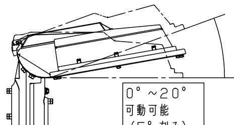
器具可動範囲
