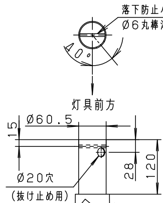
適合ポール先端形状
