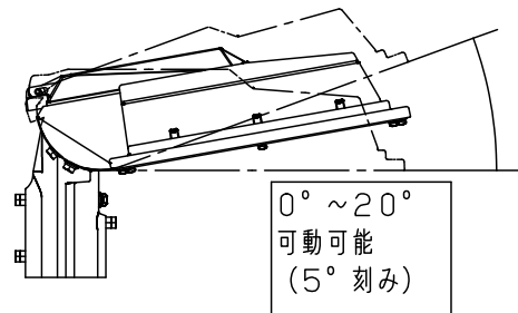
器具可動範囲
