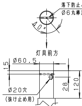
適合ポール先端形状
