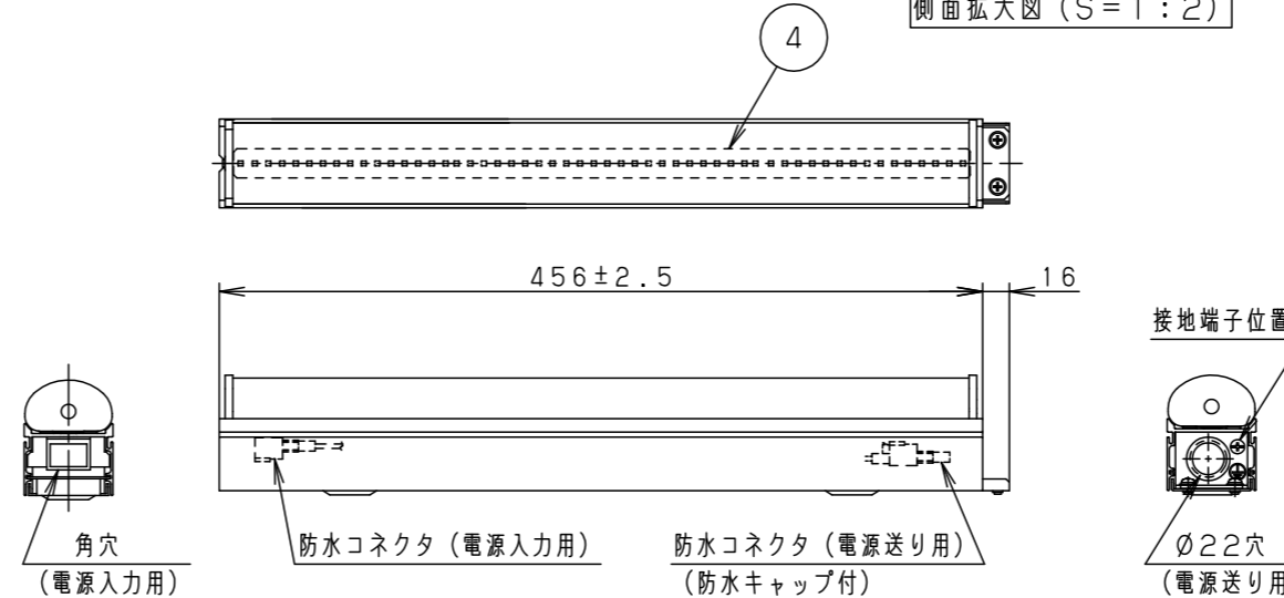
側面拡大図 (S=1:2)
