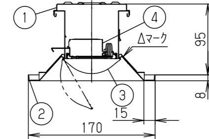
断面詳細図
