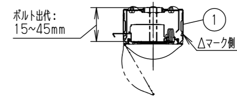
断面詳細図
