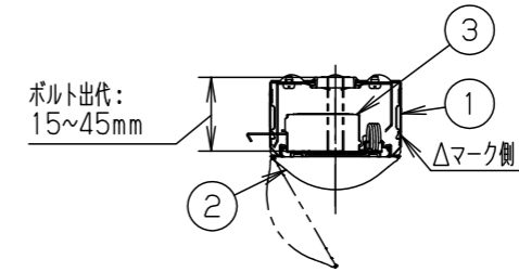
断面詳細図
