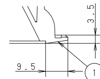
枠部詳細
