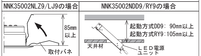
図1 埋込深さ
