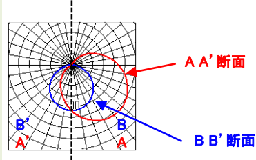
図2 配光曲線: XLX450CBLC
