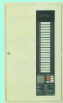
BVJ11201 20 回線埋込型内器 タテ 730 ×ヨコ 450 ×奥行 64.6
