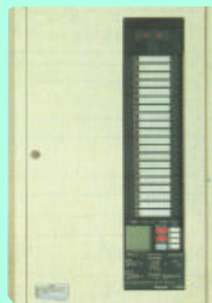
BVJ1120 20 回線露出型 タテ 680 ×ヨコ 450 ×奥行 90
