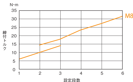
締付トルク目安※1
