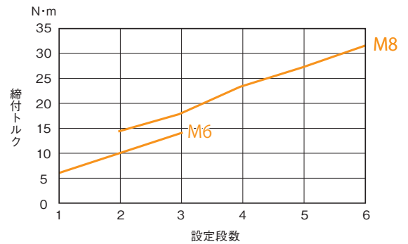
締付トルク目安*1
