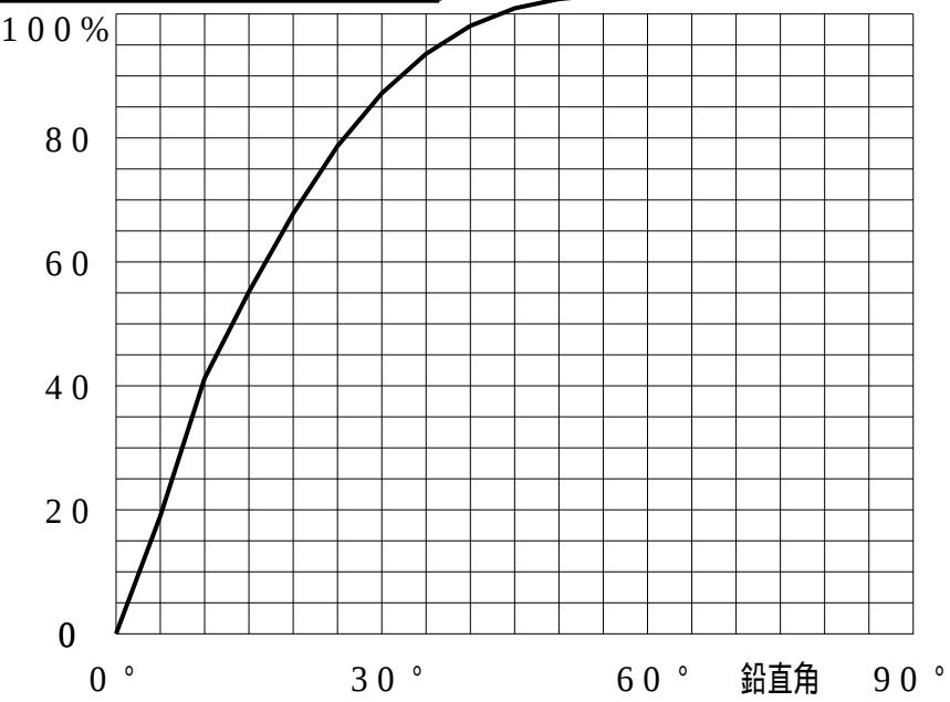
等光度曲線
