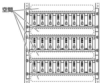
図. 19インチラックに本製品3台取付時
