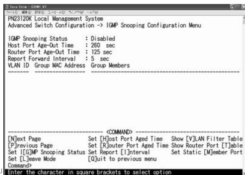
図4-7-52 IGMP Snoopingの設定
