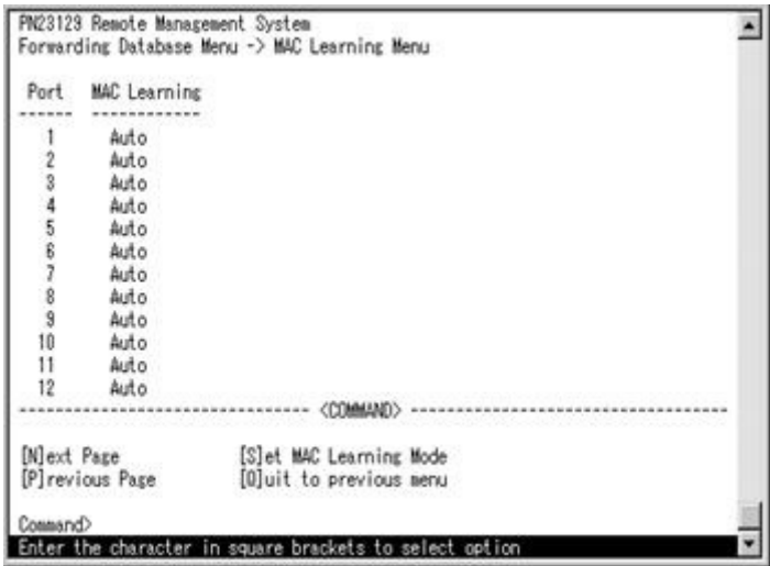
図4-6-17 ポート毎のMACアドレスの学習モードの設定
