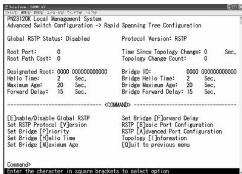
図4-7-12 スパニングツリーの設定
