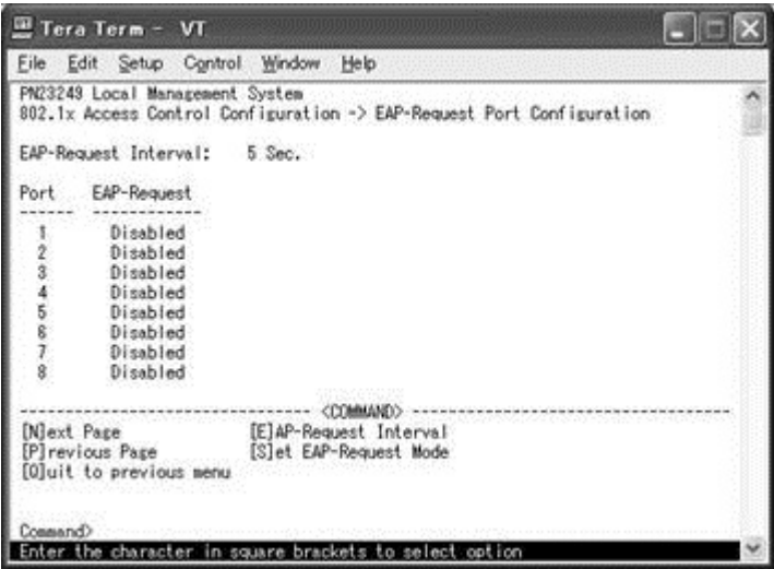
図4-7-50 EAP-Requestの送信設定
