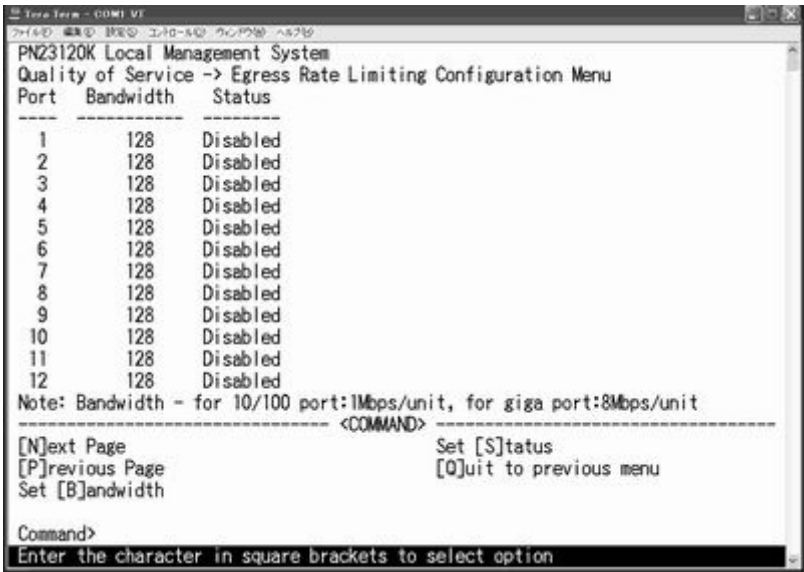
図4-7-31 帯域幅の制御設定
