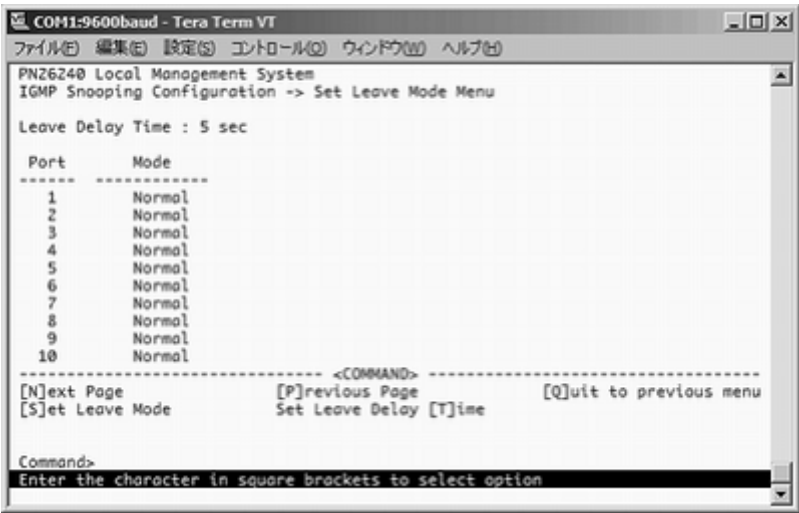
図4-7-53 Leaveモードの設定
