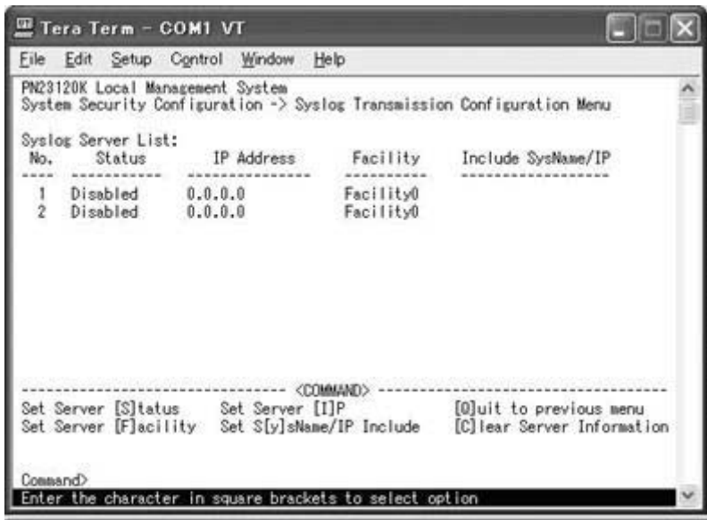
図4-6-12 Syslog Transmissionの設定
