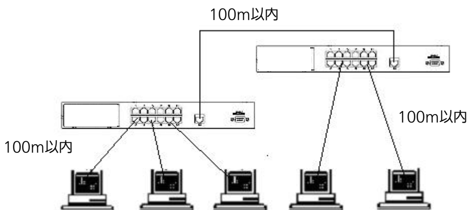
図3-1 接続構成例
