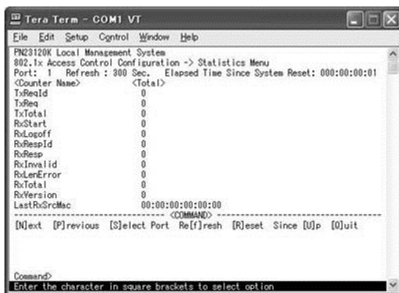
図4-7-48 カウンタクリアからの累積表示
