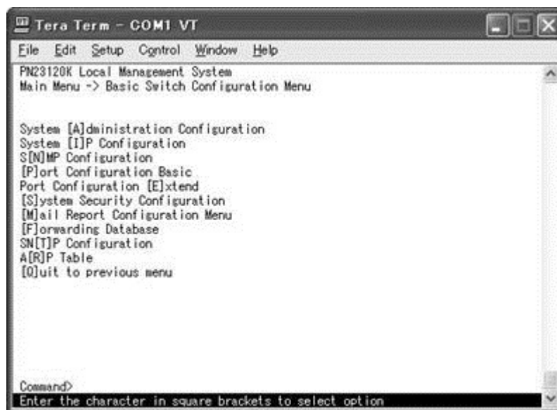
図4-6-1 スイッチの基本機能設定メニュー
