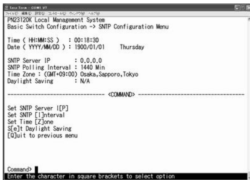
図4-6-21 時刻同期機能の設定：設定前
