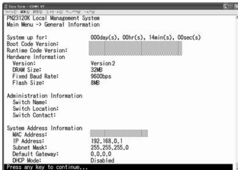
図4-5-1 基本情報の表示
