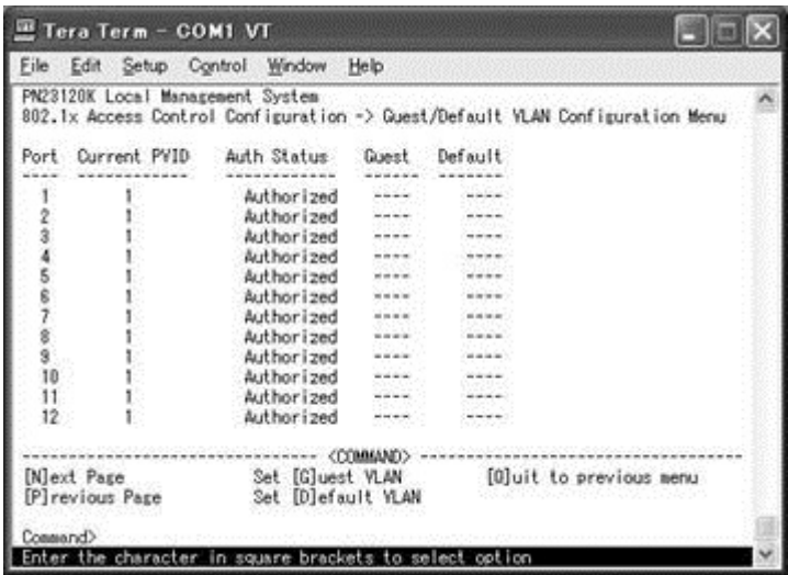
図4-7-37 Guest/Default VLANの設定
