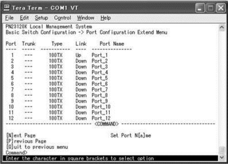
図4-6-9 各ポートの設定
