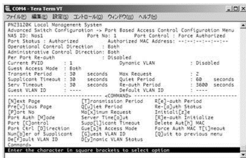
図4-7-34 IEEE802.1Xポートベース認証機能の設定
