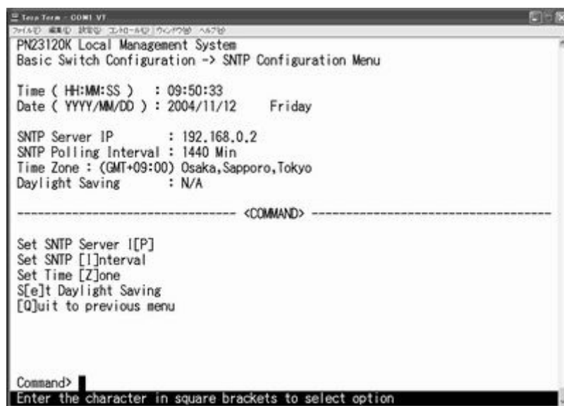
図4-6-22 時刻同期機能の設定：設定後
