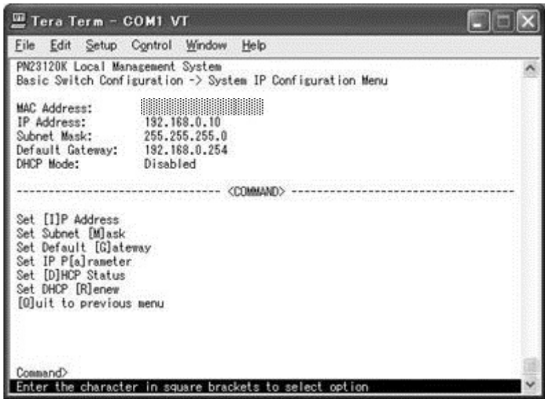
図4-6-3 IPアドレスの設定
