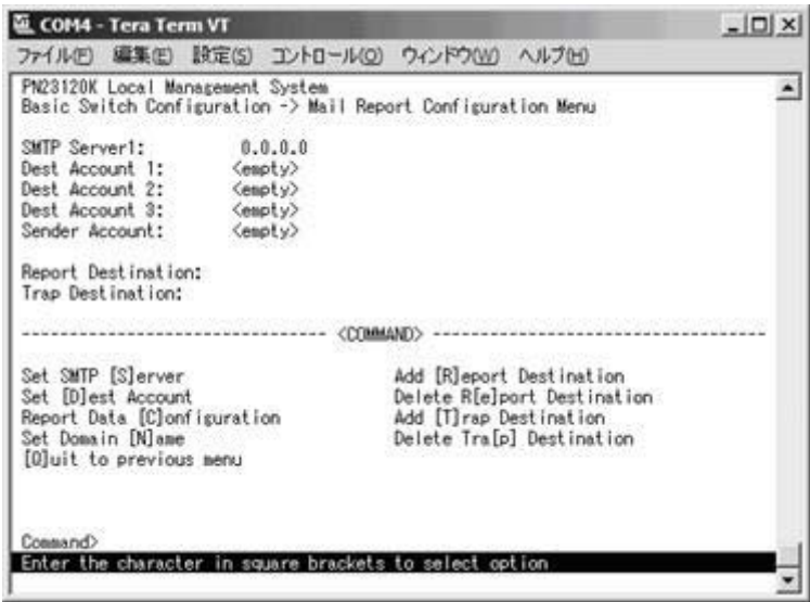
図4-6-13 E-mail通知機能の設定
