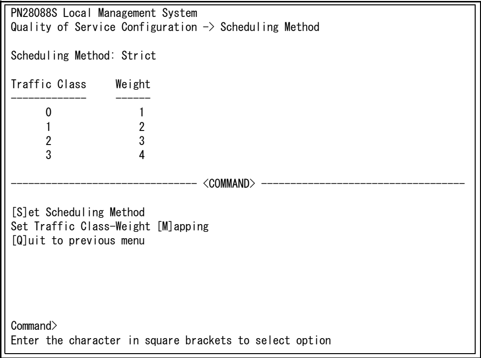
図 4-6-5-3 スケジューリング方式の設定
