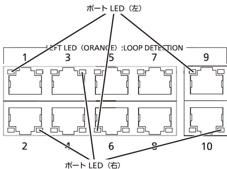
図 1-2 ポート LED
