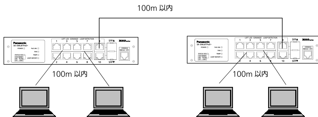
図 3-1 接続構成例
