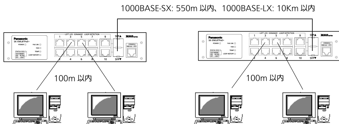
図 3-2 光ファイバケーブル接続例
