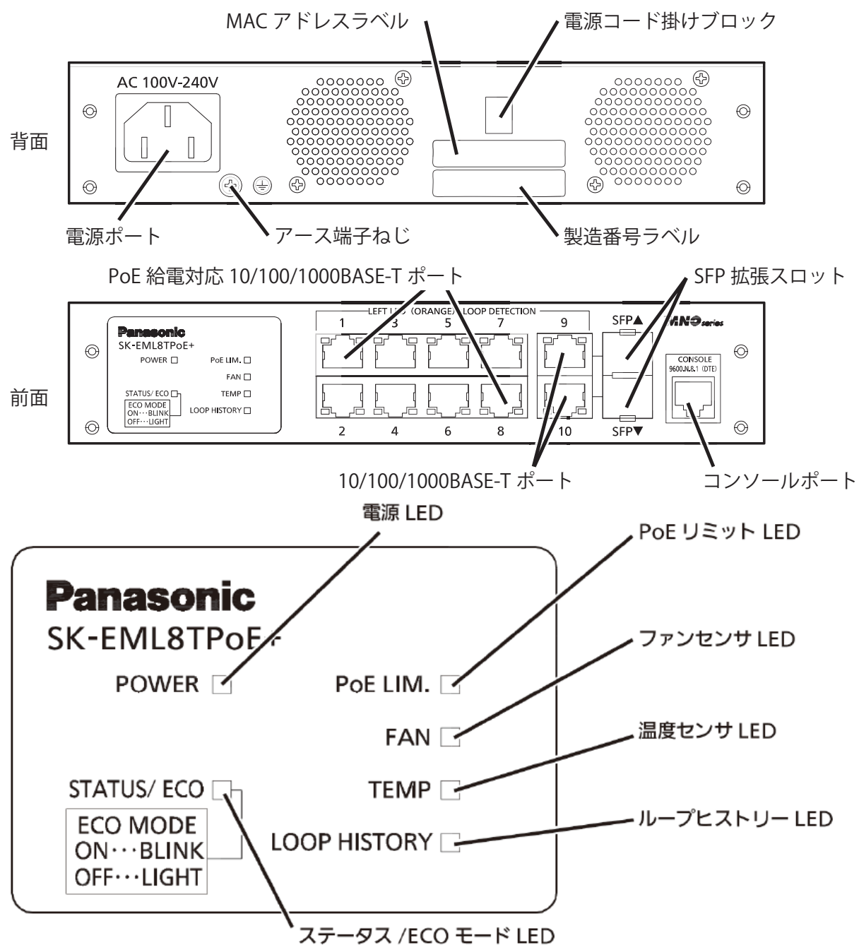
図 1-1 各部の名称
