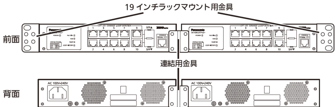
図 2-2 ラックへの設置
