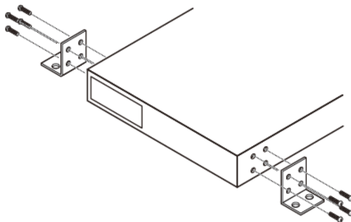
図 2-3 壁面への設置
