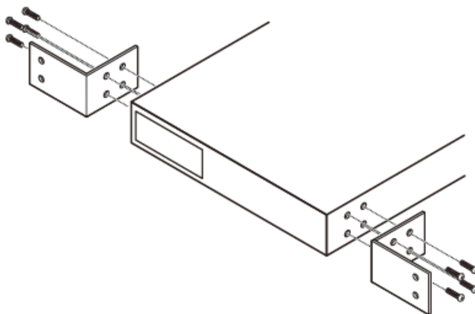
図 2-2 ラックへの設置
