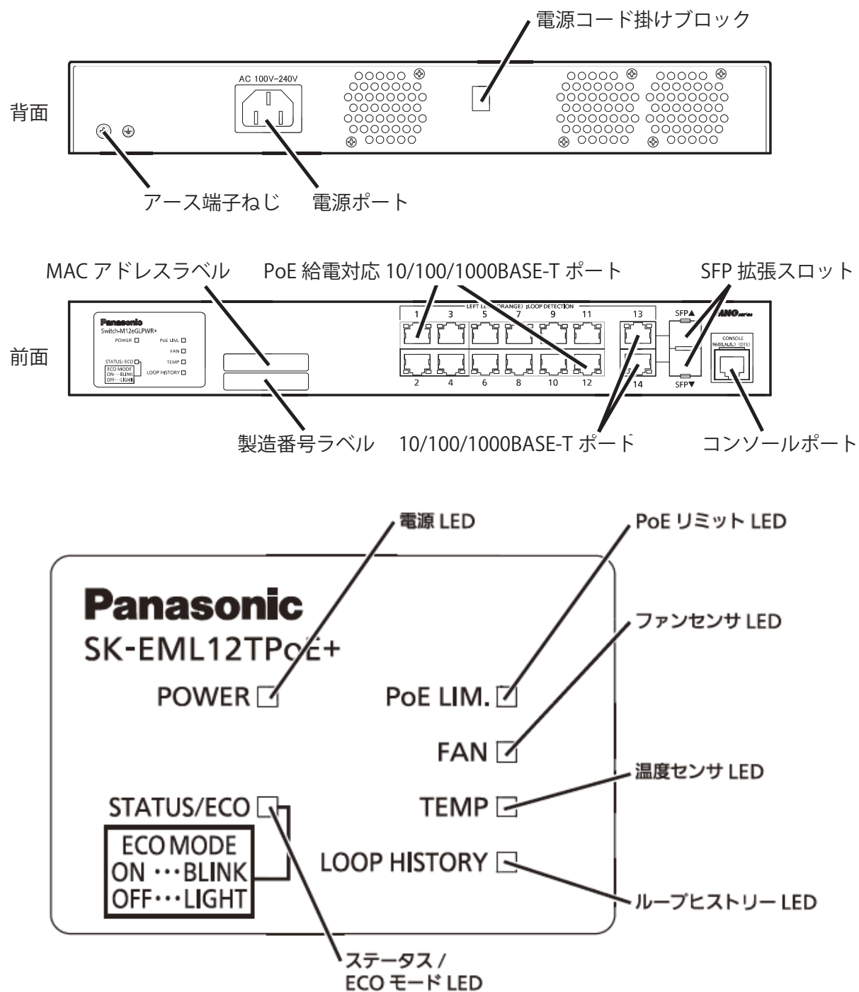
図 1-1 各部の名称
