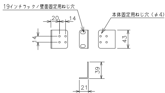
19インチラックノ壁面固定用金具 (同梱)
