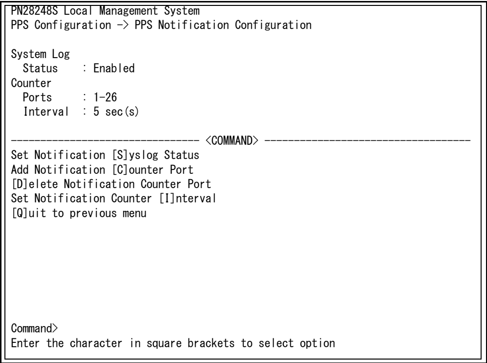
図 4-6-12-2 PPS 通知設定
