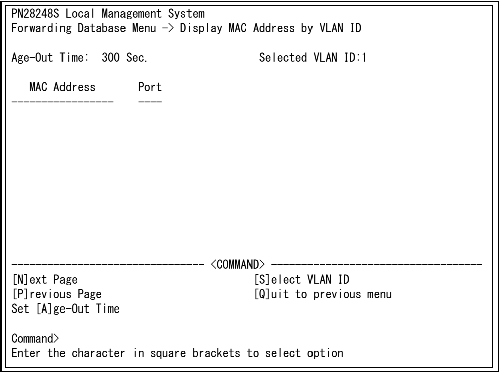
図 4-5-8-6 VLAN 毎の MAC アドレステーブルの表示
