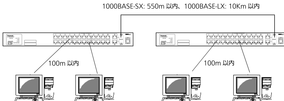
図 3-2 光ファイバケーブル接続例
