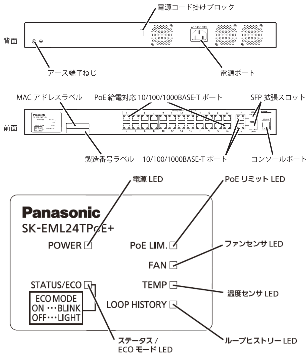
図 1-1 各部の名称
