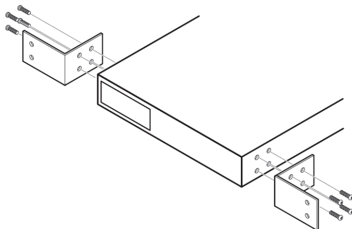
図 2-1 ラックへの設置
