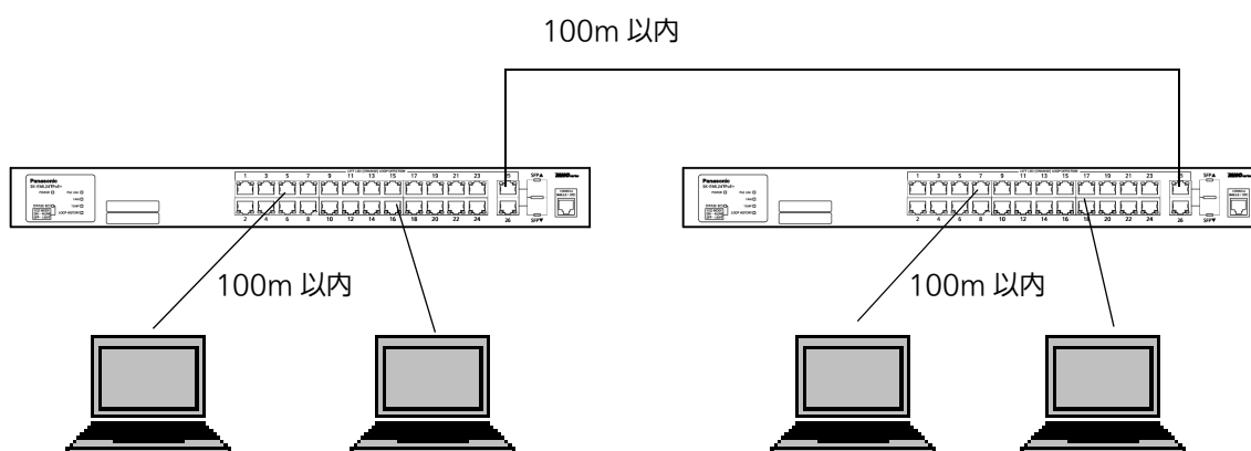
図 3-1 接続構成例
