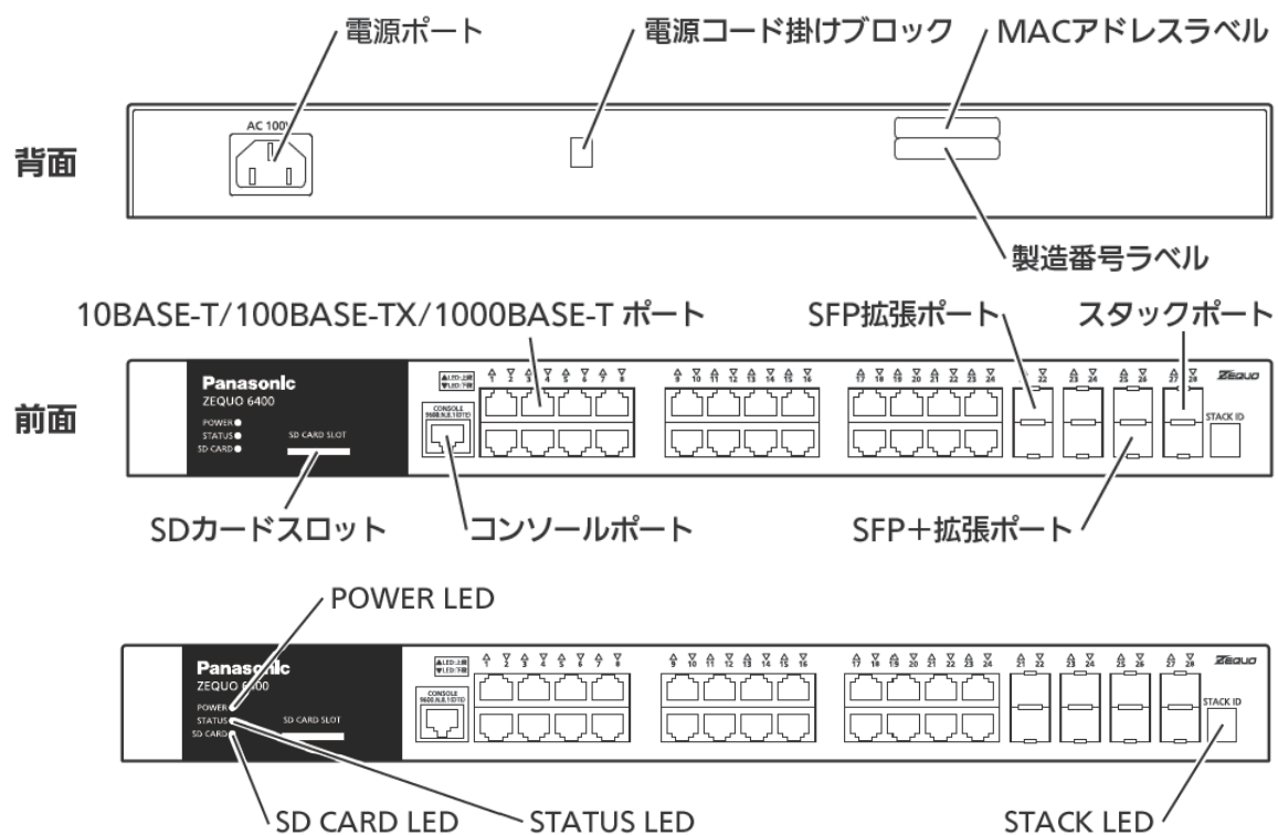
図 1-1 背面、前面、LED
