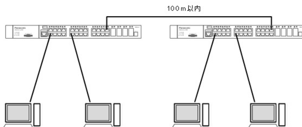
図 3-1 接続構成例
