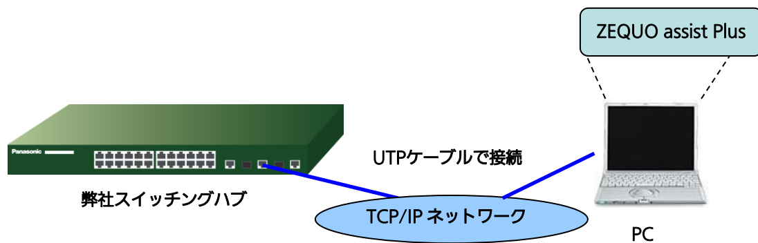
図 7-1-2 接続構成図(Telnet/SSH 経由)
