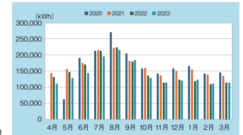
倉敷中島店における電力量の推移
