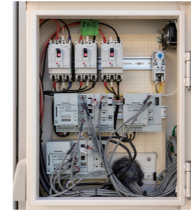
多回路エネルギーモニタ
