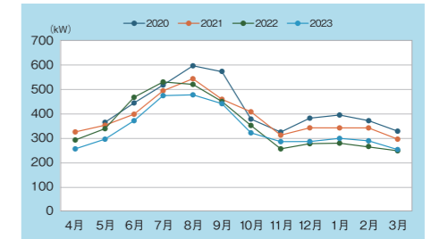
倉敷中島店における最大需要電力(デマンド値)の推移
