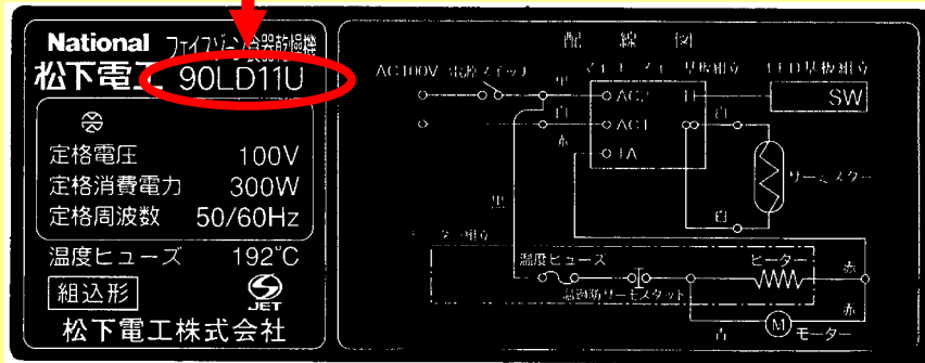
定格銘板・回路図
