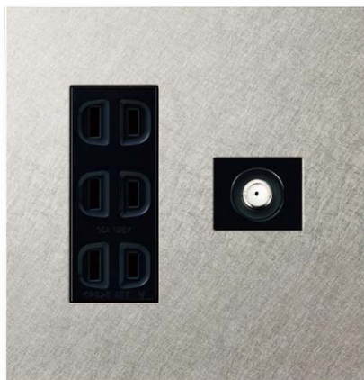
コンセント:WTL13033B TVコンセント:WCS3013B プレート:WNS9674S 取付枠:WTL3710K
