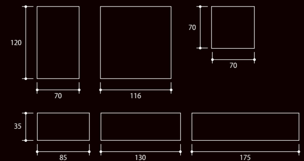
プレート外形寸法 寸法表示単位:mm
