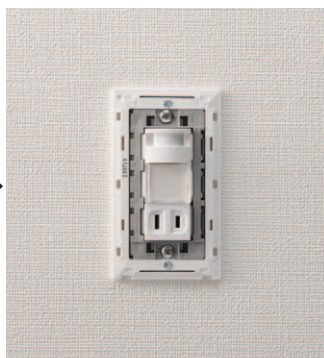
プレート枠を取りつける。
