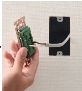
コンセントを取り出す。
