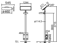
■ポール底面取付寸法図
