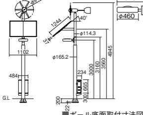
■ポール底面取付寸法図
