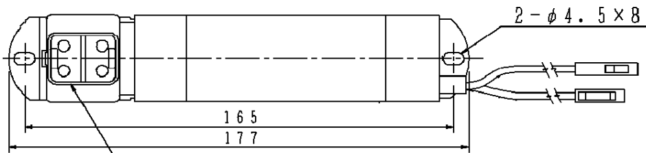
電源接続用端子台 (送り付 20A以下)
